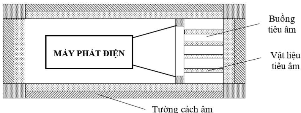
Hình 4.4. Sơ đồ nguyên lý buồng tiêu âm chống ồn
