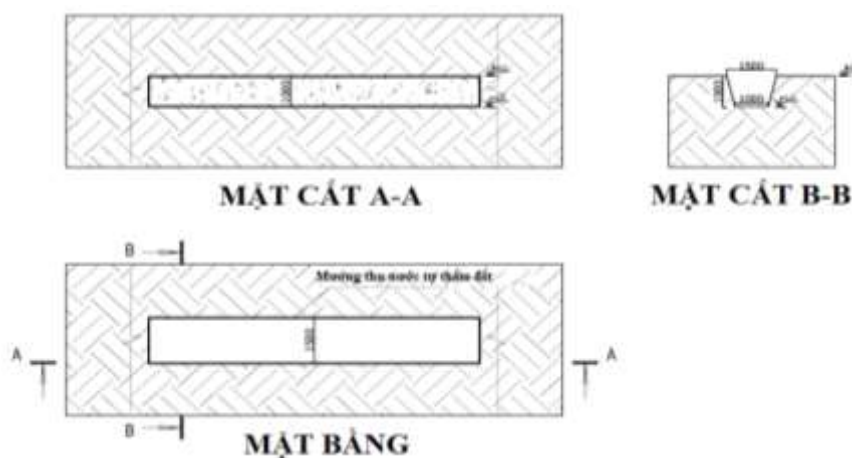
Hình 3.4. Sơ đồ dự kiến tuyến mương tạm thu gom nước mưa trong giai đoạn thi công
