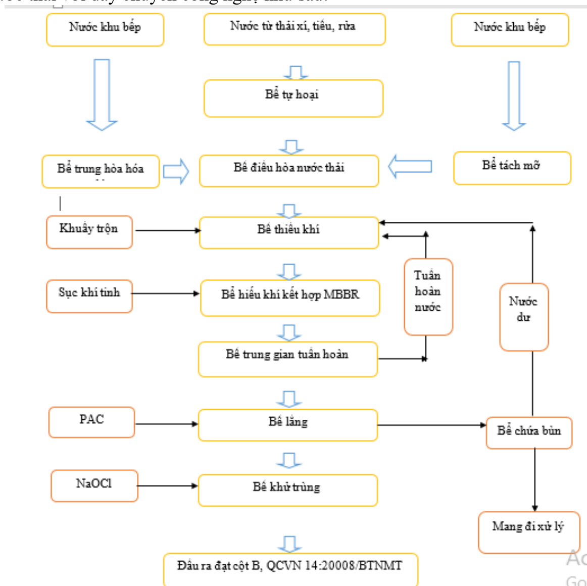
Sơ đồ dây chuyền công nghệ
