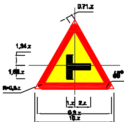
Biển số W.205b: Đường giao nhau
