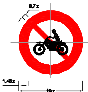
Biển số P.104: Cấm xe mô tô
