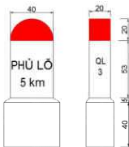
Hình I.1 - Cột kilômét dạng cột thấp
