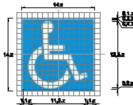
Biển số 1.446 : Nơi đỗ xe dành cho người khuyết tật
