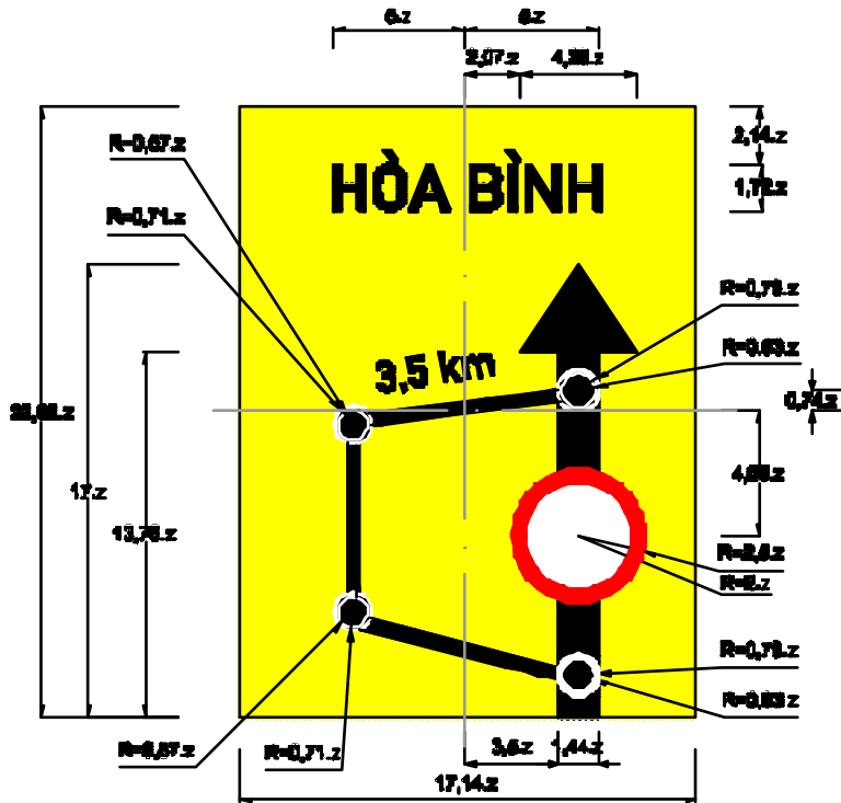
Biển số 1.416 : Đường tránh
