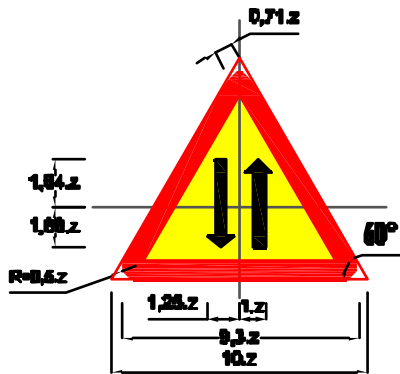
Biển số W.204: Đường hai chiều
