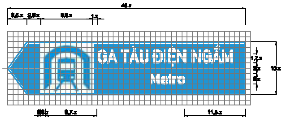
Biển số L44k : Biển báo chỉ dẫn địa điểm
