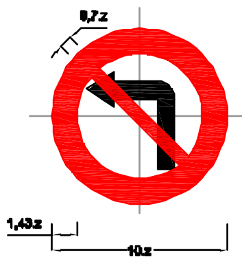
Biển số P.123a: Cấm rẽ trái
