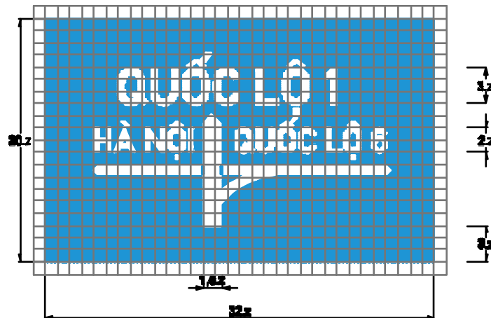
Biển số 1.447b: Biển báo cầu vượt lên thông
