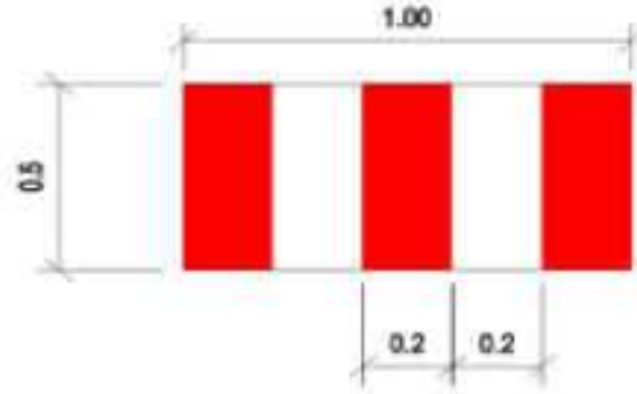
Hình G.65 - Chi tiết vạch 8.2
