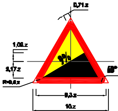
Biển số W.220: Đốc lên nguy hiểm
