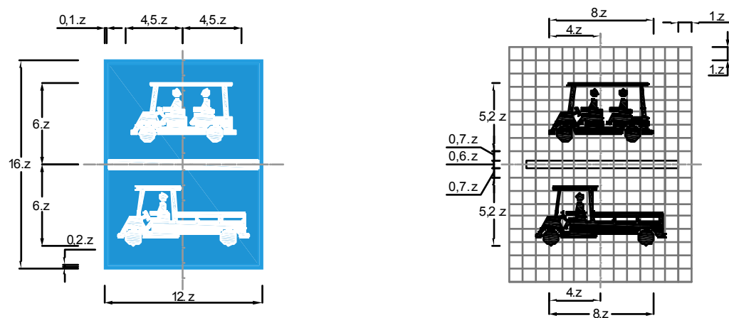
Biển số R.403k: Đường dành cho xe chở hàng, xe chở người bốn bánh gắn động cơ
