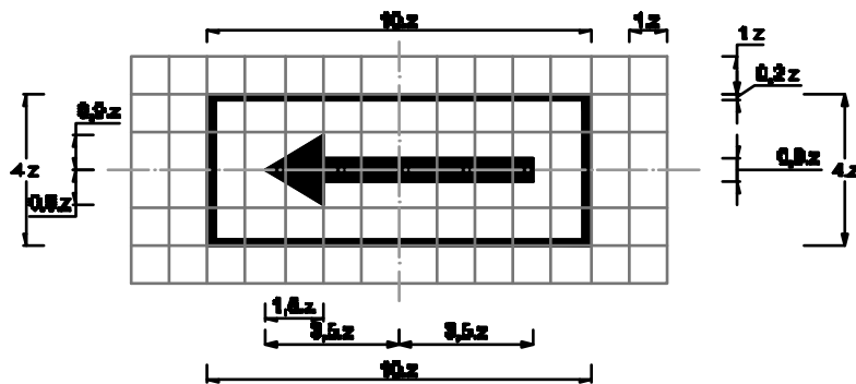
Biến số S.503d: Hướng tác dụng của biến
