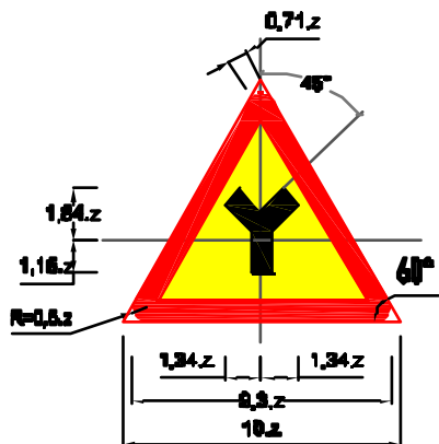
Biển số W.205e: Đường giao nhau
