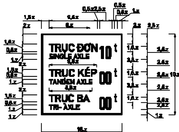
Biển số 5.505c : Tải trọng trục hạn chế qua cầu
