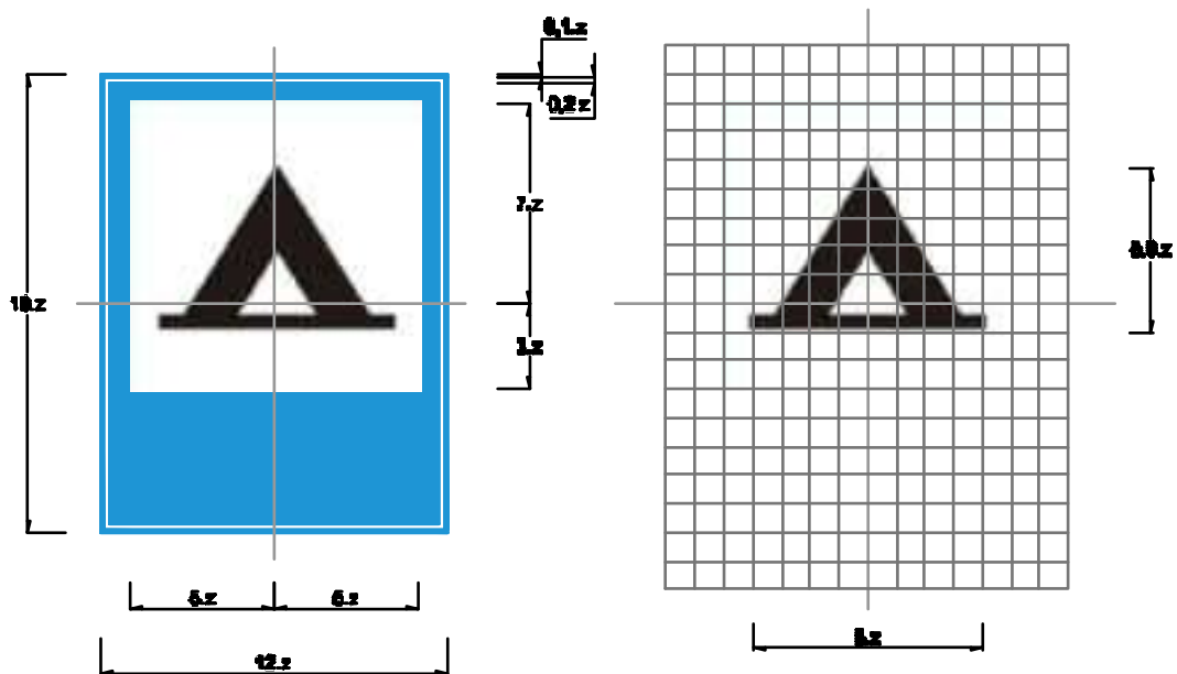
Biển số L433b : Báo hiệu nơi cắm trại, nhà nghỉ lưu động
