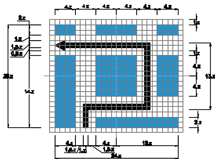
Biển số I.418a : Chỉ dẫn địa giới 34z (Thay đổi tùy theo số lượng chữ)
