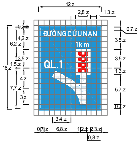
Biển số I.448 : Làn đường cứu nạn hay làn thoát xe khẩn cấp
