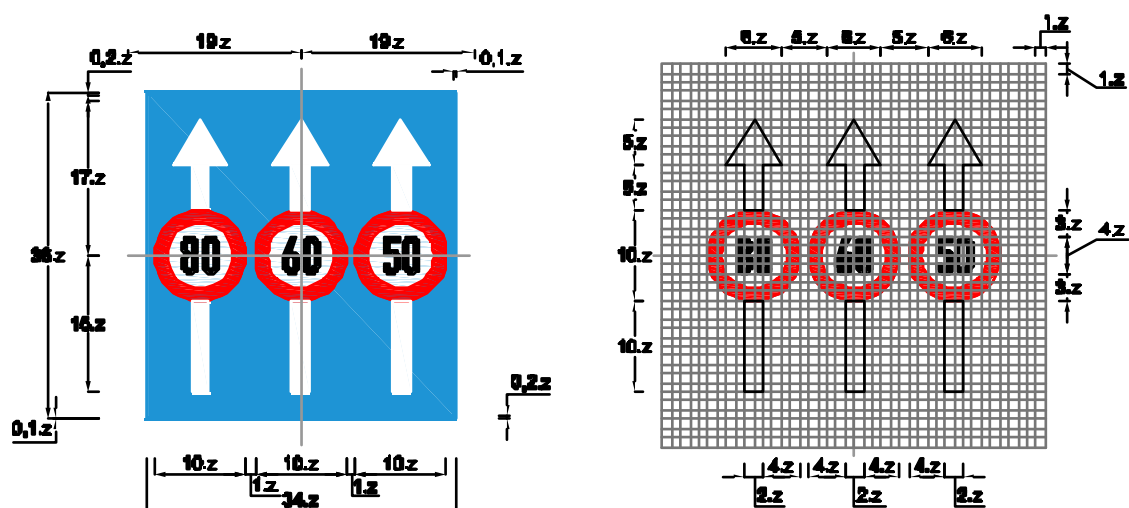
Biển số P.127b: Biển gộp tốc độ tối đa cho phép theo làn đường đặt bên đường hoặc trên cột cần vươ
