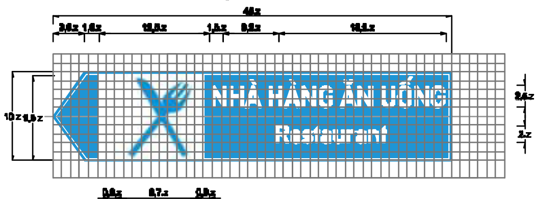
Biển số L44l : Biển báo chỉ dẫn địa điểm
