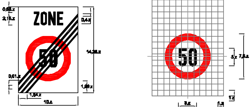
Biển số R.E,10c: Hết hạn chế tốc độ tối đa trong khu vực
