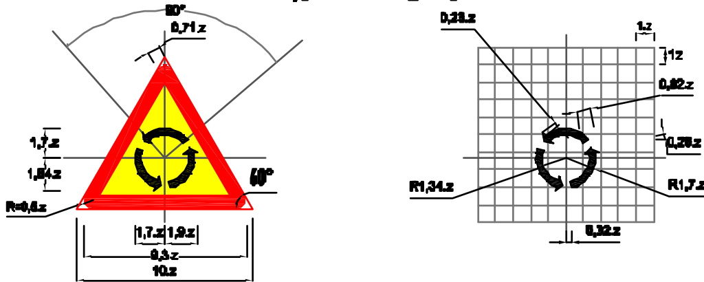
Biển số W.206: Giao nhau theo vòng xuyến
