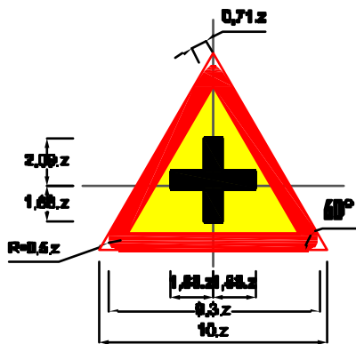
Biển số W.205a: Đường giao nhau
