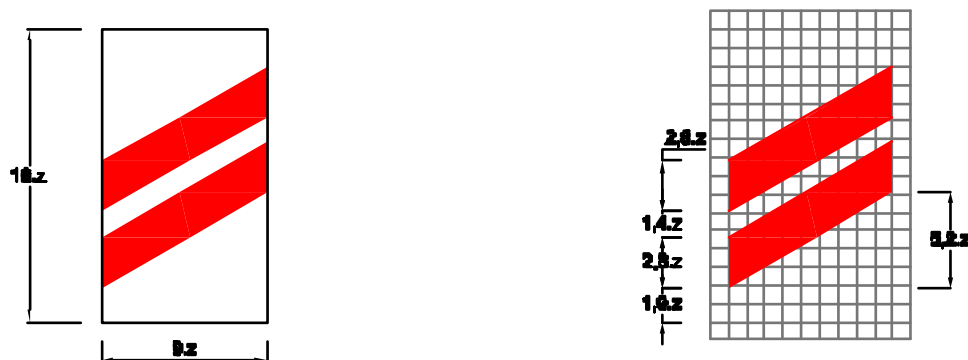
Biên số W.243b: Nơi đường sắt giao không vuông góc với đường bộ
