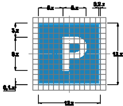
Biển số L408a : Nơi đỗ xe một phần trên hè phố
