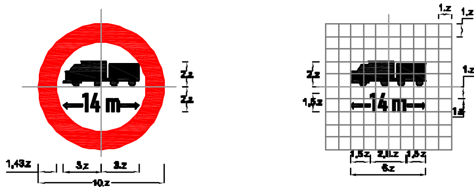
Biển số P.120: Hạn chế chiều dài xe ô tô, máy kéo moóc hoặc sơ-mi-rơ moóc
