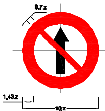
Biển số P.136: Cấm đi thẳng
