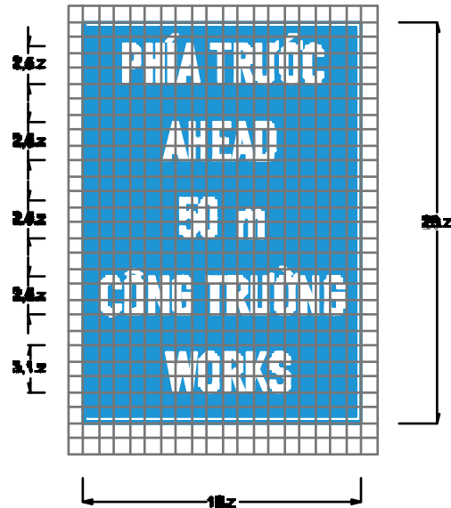
Biển số L441c : Biển hiệu phía trước số công trường thi công
