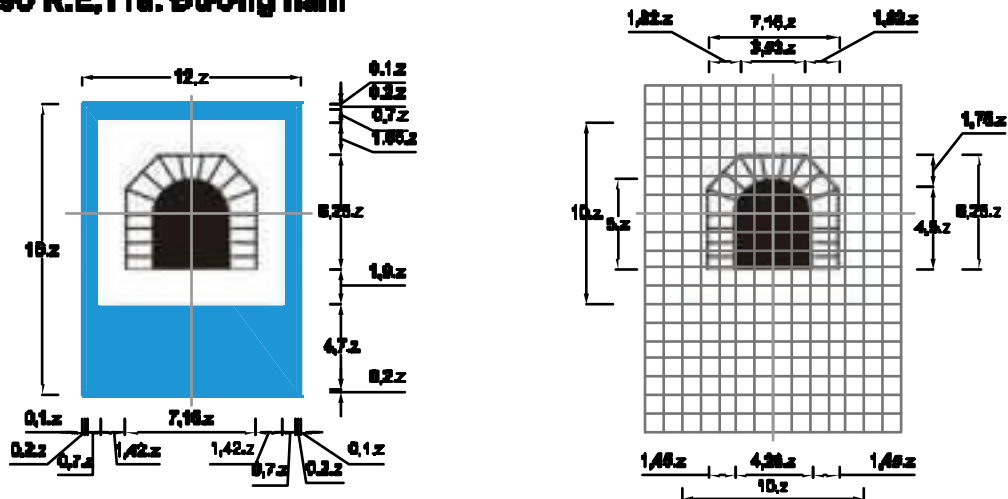
Biển số R.E,11b: Hết đường hầm
