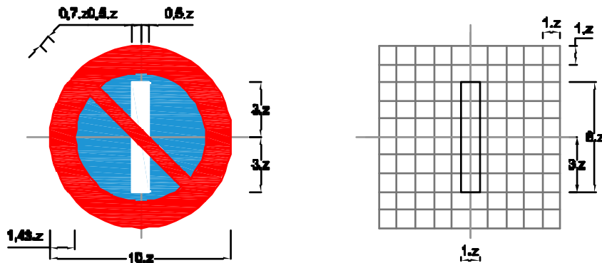
Biển số P.131b: Cấm đỗ xe vào ngày lễ
