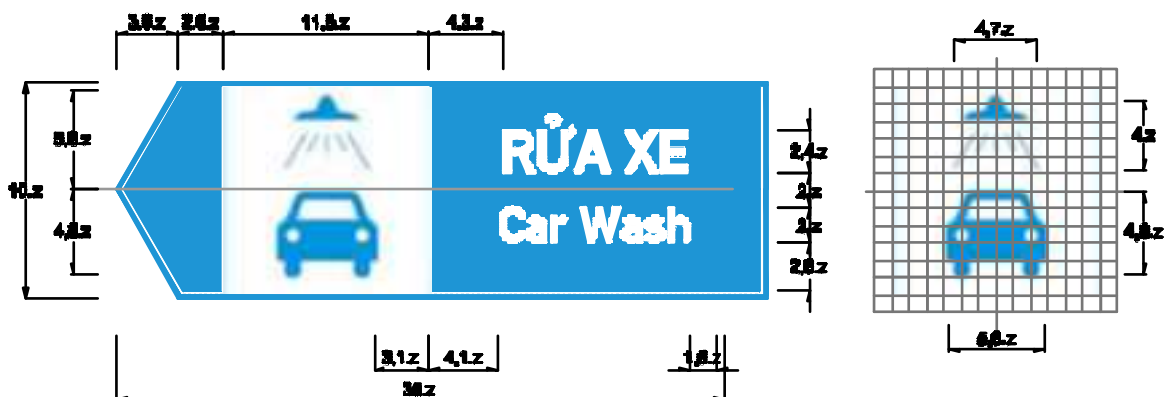
Biển số L.444i : Biển báo chỉ dẫn địa điểm
