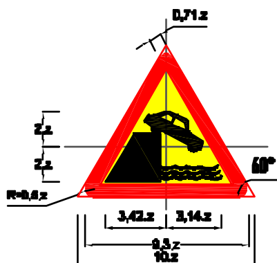
Biển số W.215a: Kè, vệt sâp phía trước
