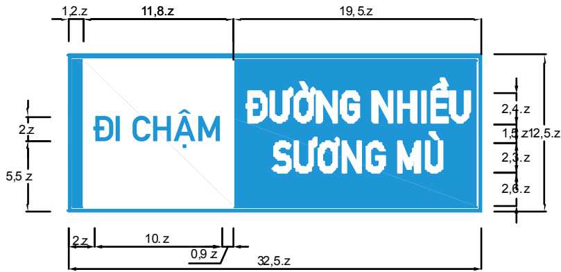
Biển số I.445c: Biển báo mô tả tình trạng đường
