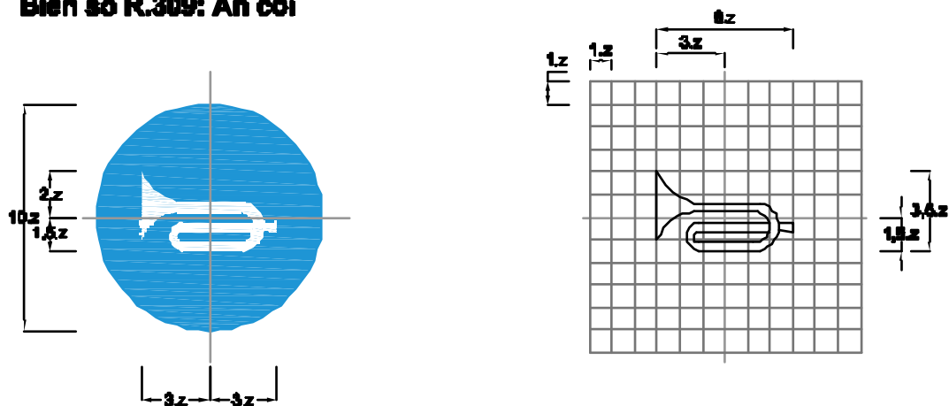
Biển số R.309: Ấn còi
