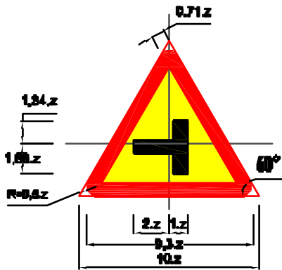
Biển số W.205c: Đường giao nhau
