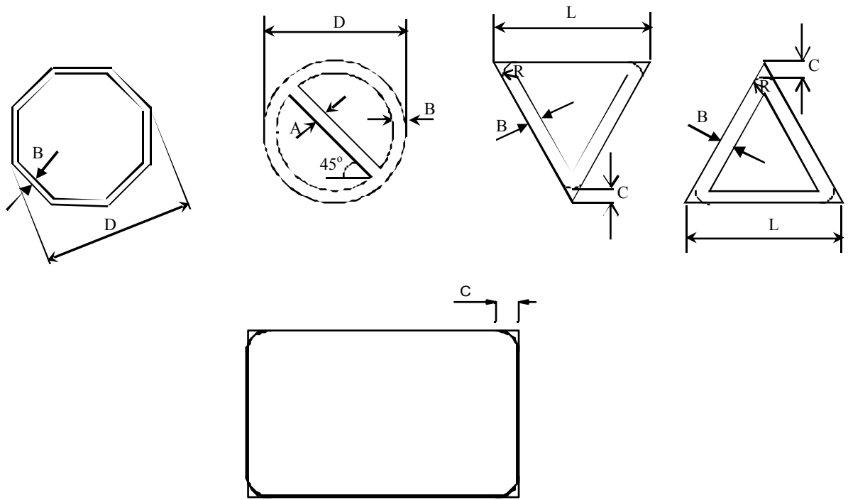
Hình 1 - Kích thước các loại biển báo
