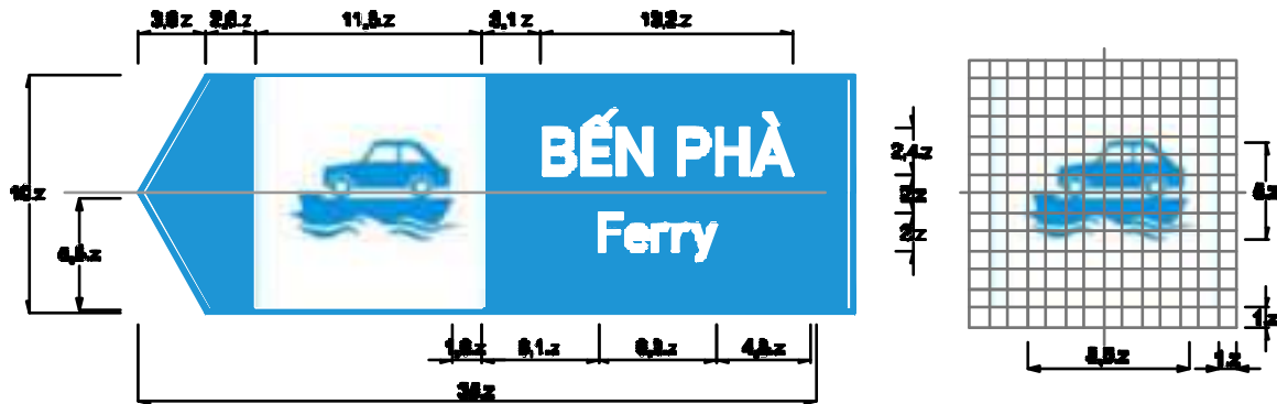
Biển số L44j : Biển báo chỉ dẫn địa điểm
