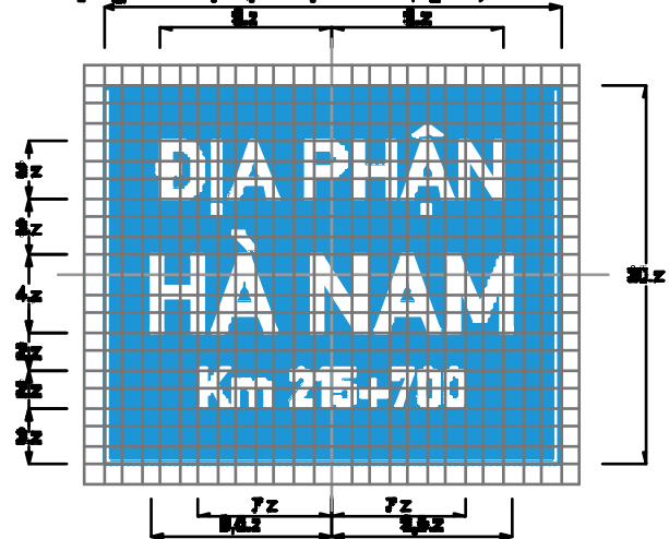
Biển số I.418b : Chỉ dẫn địa giới trên tuyến đường đối ngoại
