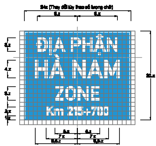
Biển số I.418b : Chỉ dẫn địa giới trên tuyến đường đối ngoại
