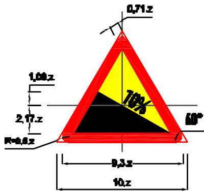
Biển số W.219: Đốc xuống nguy hiểm
