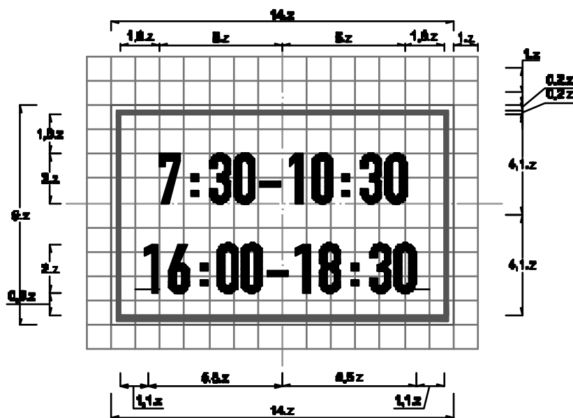
Biển số S.508b : Biểu thị thời gian
