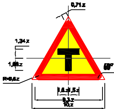
Biển số W.205d: Đường giao nhau
