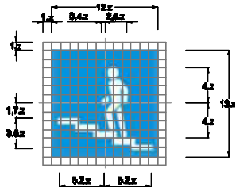
Biển số L424b : Cầu vượt qua đường cho người đi bộ
