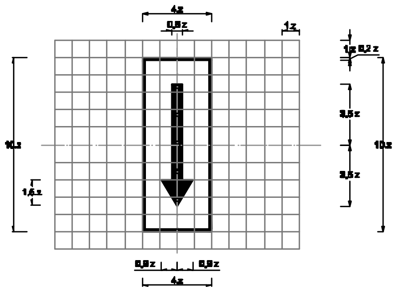
Biến số S.503d: Hướng tác dụng của biến
