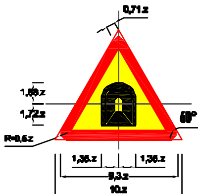
Biển số W.240: Đường hầm
