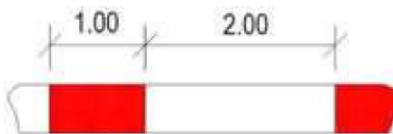
Hình G.68 - Chi tiết vạch 8.5
