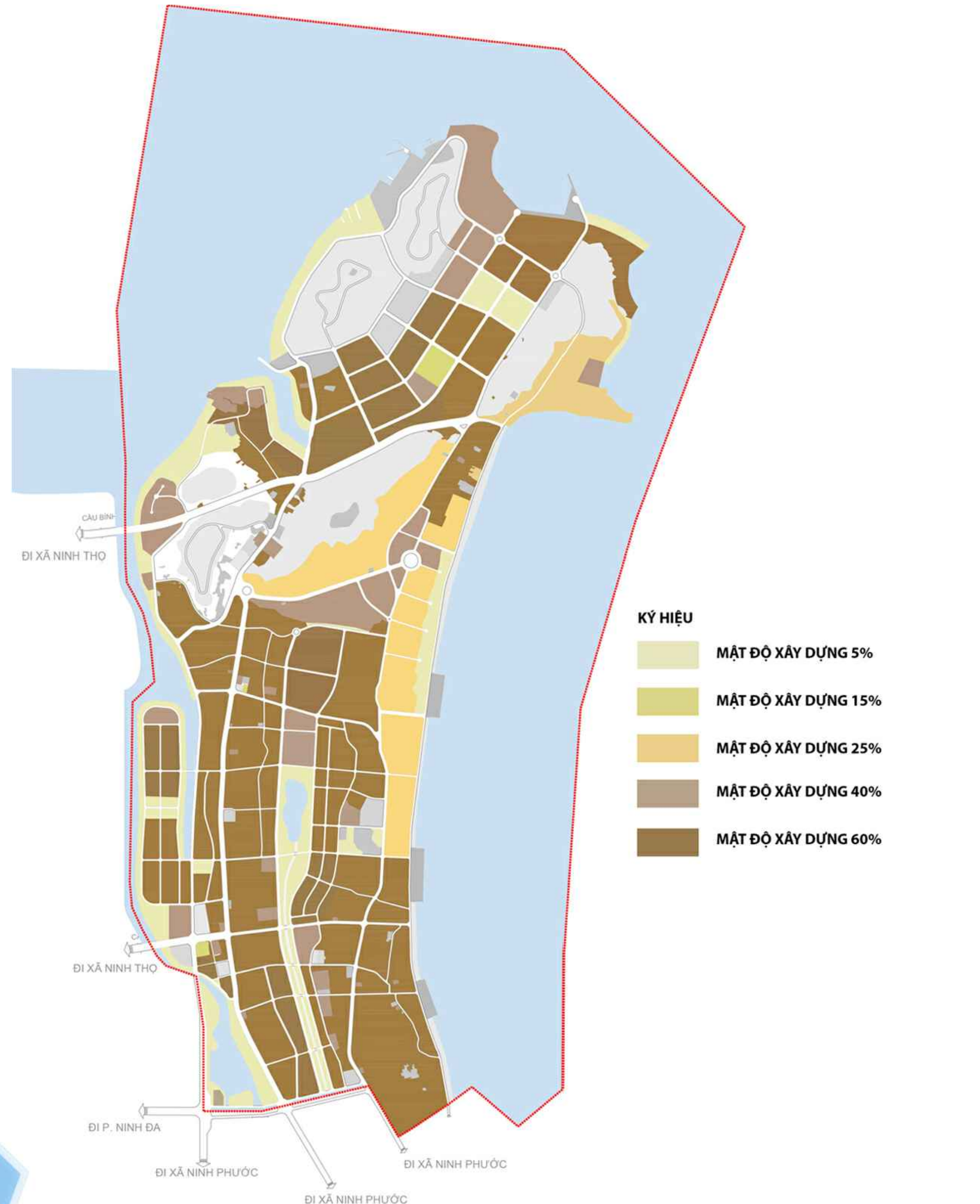
SƠ ĐỒ PHÂN BỐ MẬT ĐỘ XÂY DỰNG CÔNG TRÌNH
