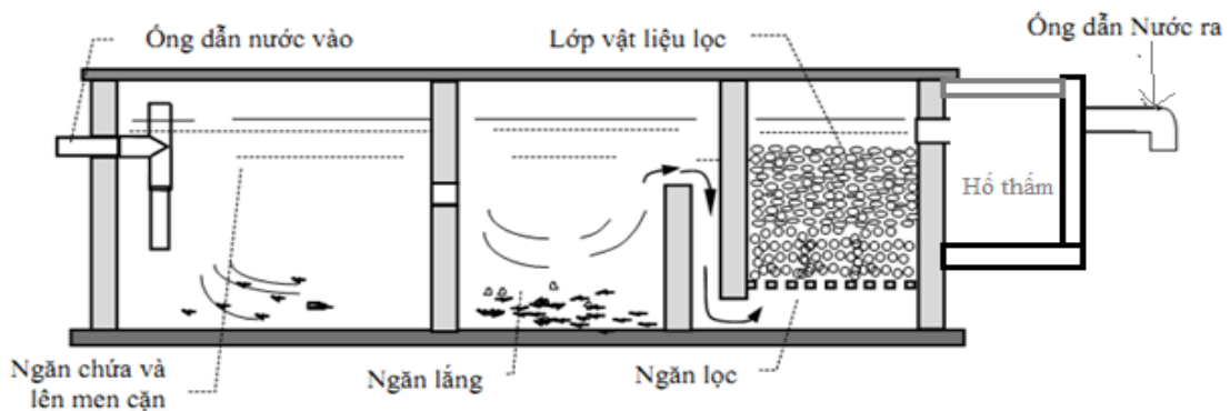
Hình 1. Mô hình hầm tự 3 ngăn
