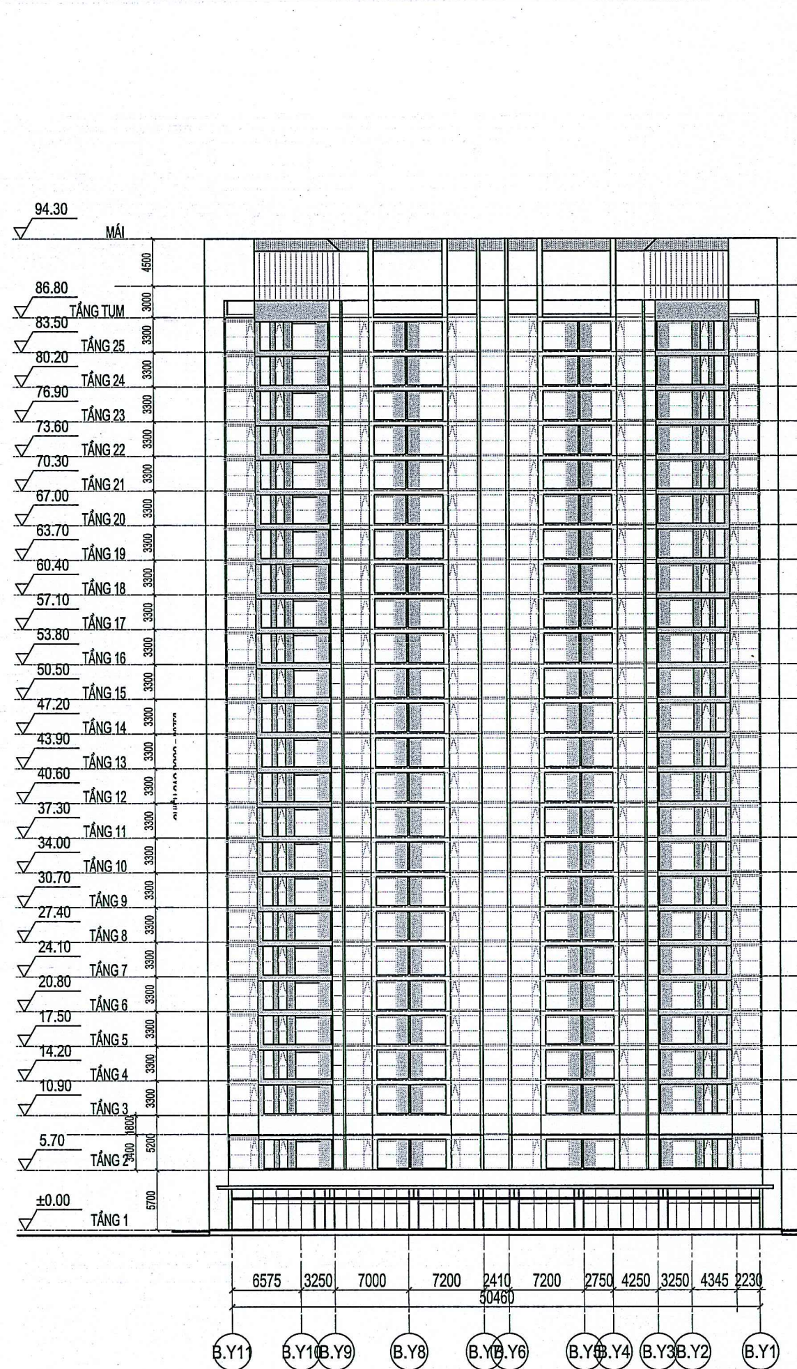
CT1 - MẶT ĐỨNG TRỤC B.Y11 - B.Y1
