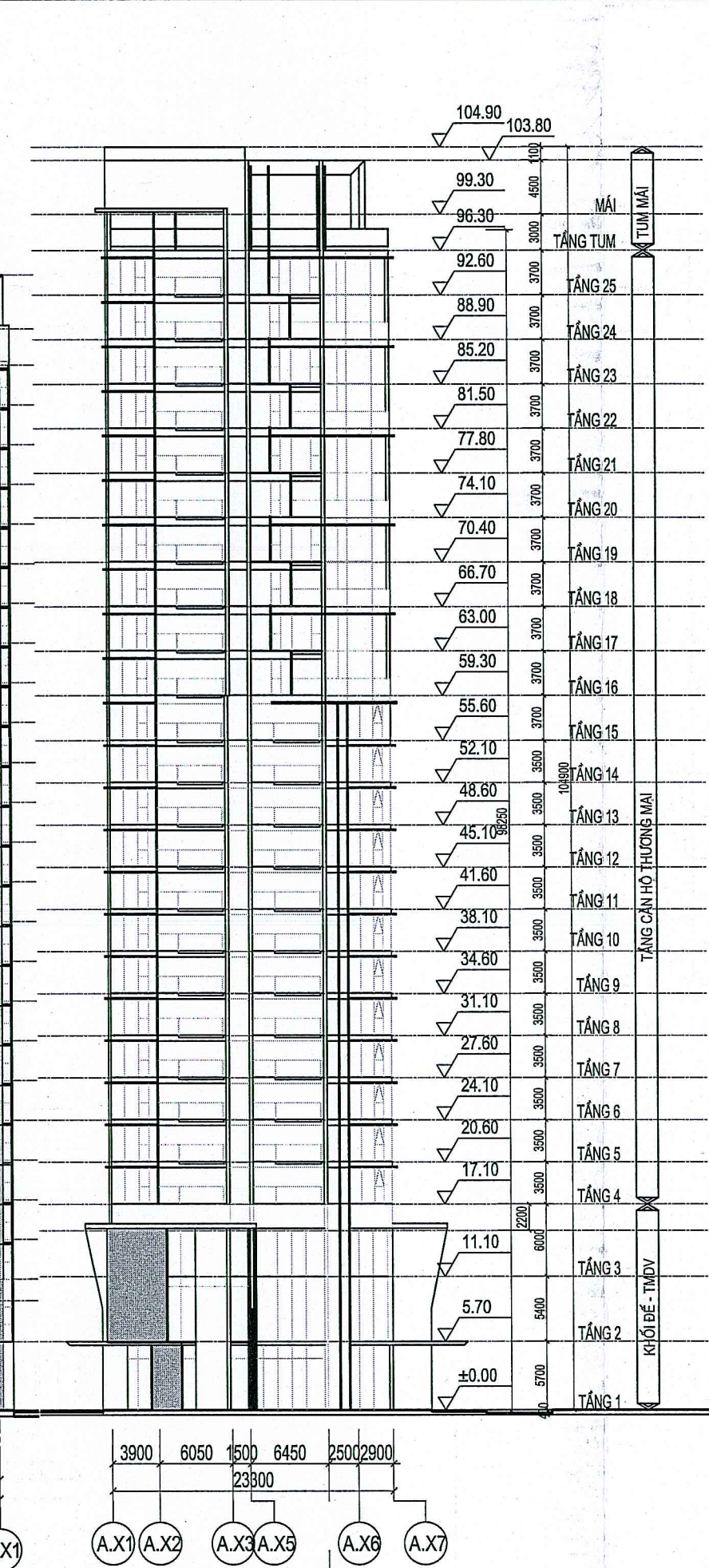
CT2 - MẶT ĐỨNG TRỤC A.X1-A.X7
