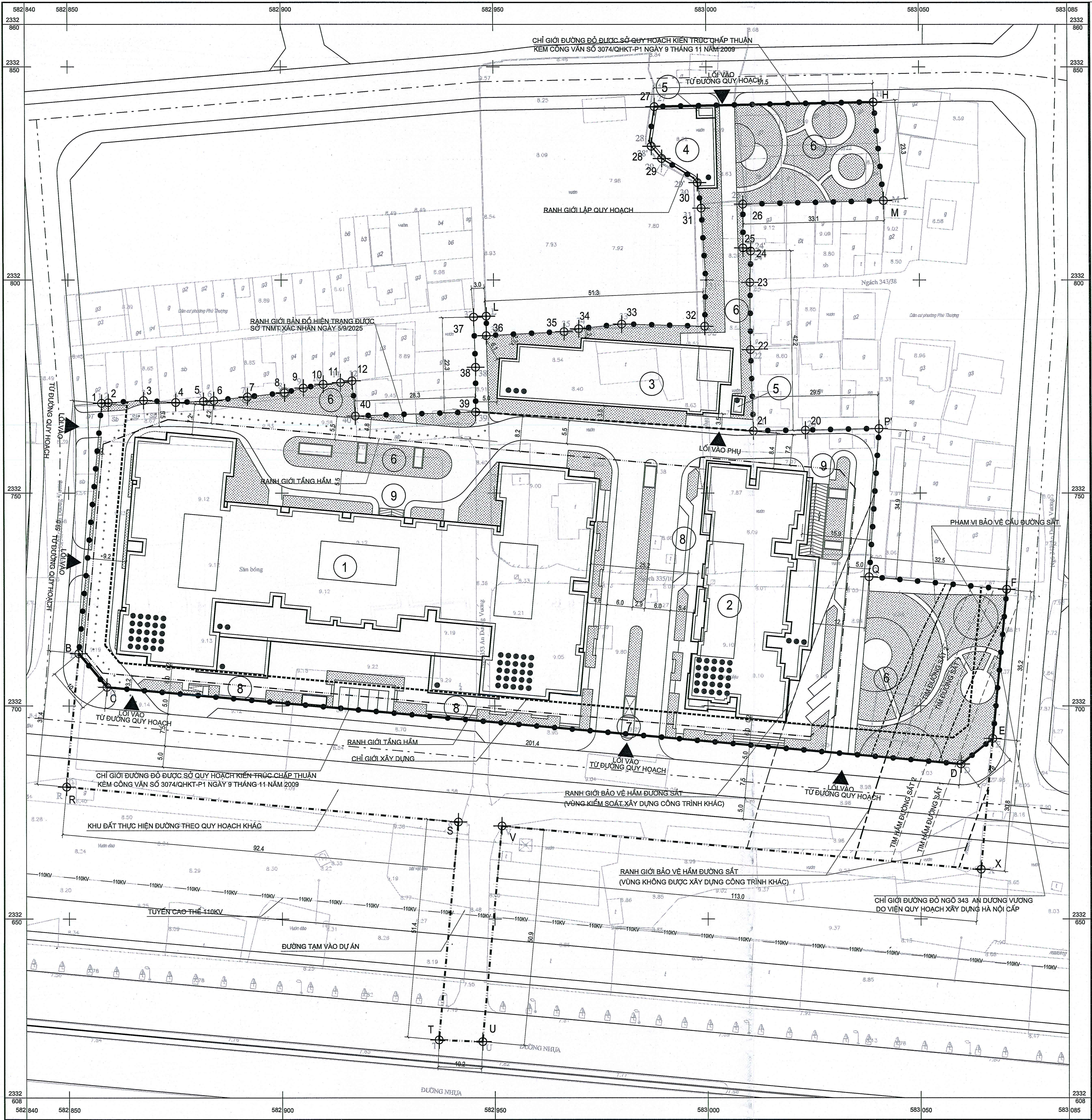
TỔNG MẶT BẰNG TỶ LỆ: 1/500
