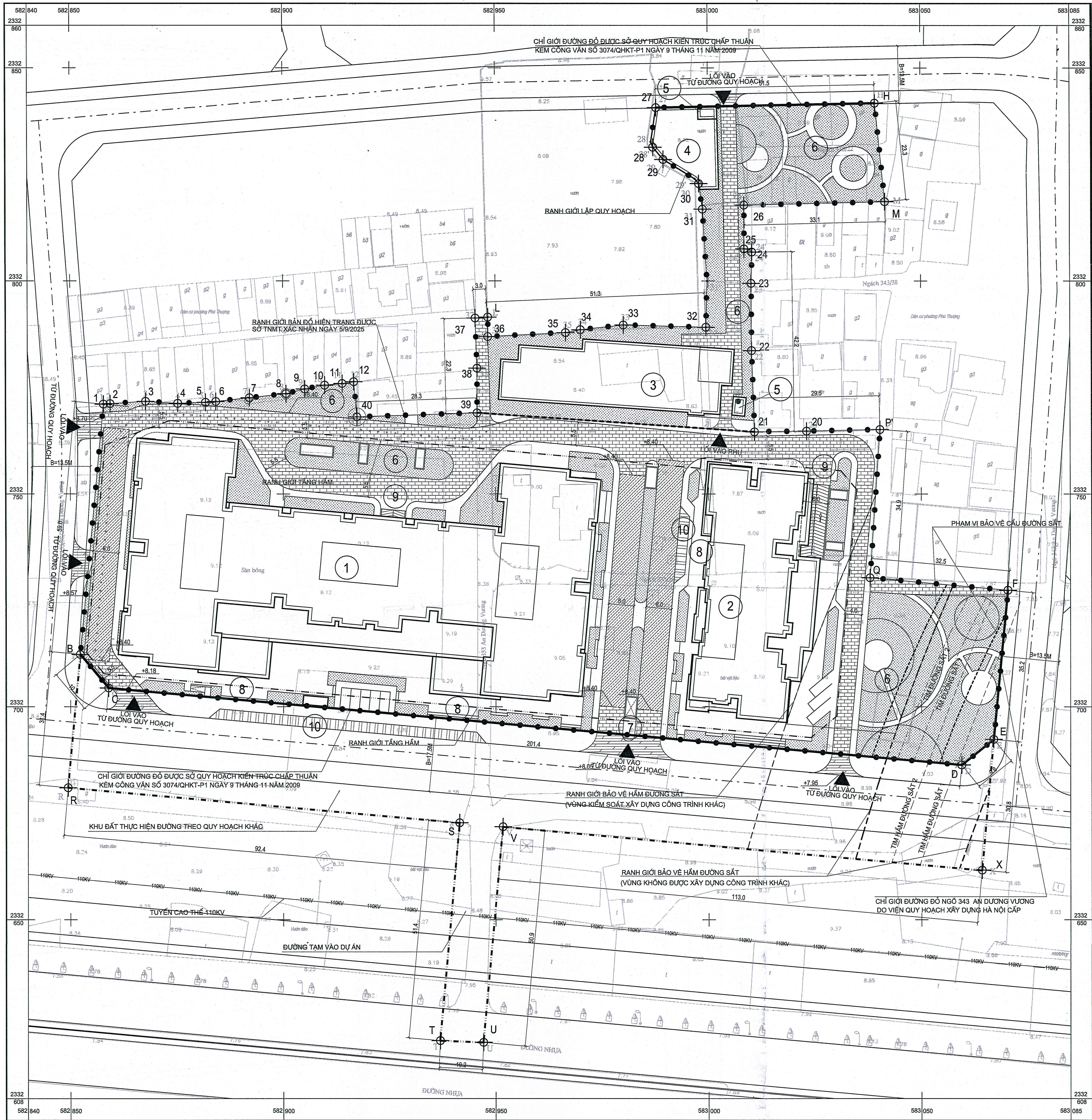
TỔNG MẶT BẰNG GIAO THÔNG TỶ LỆ: 1/500
