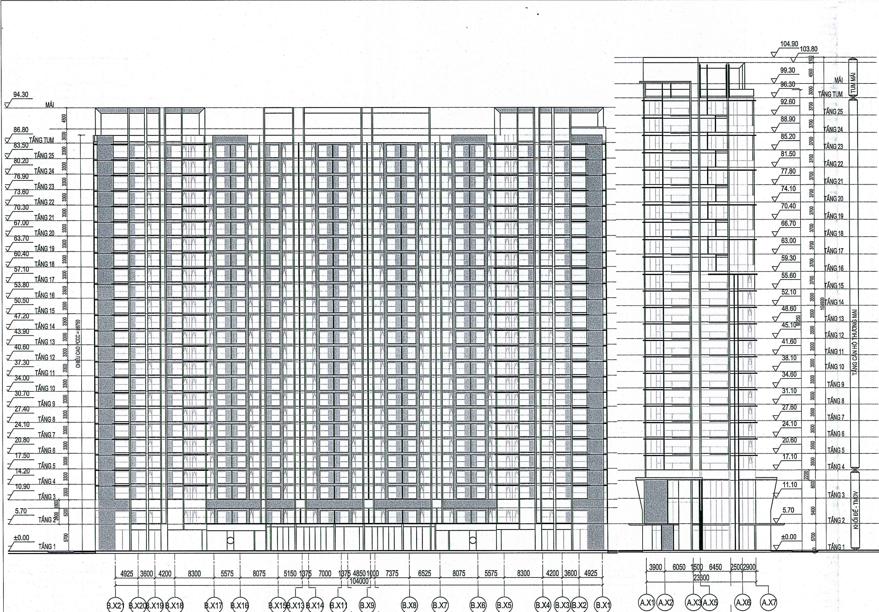
CT1-MẶT ĐỨNG TRỤC B.X21- B.X1
