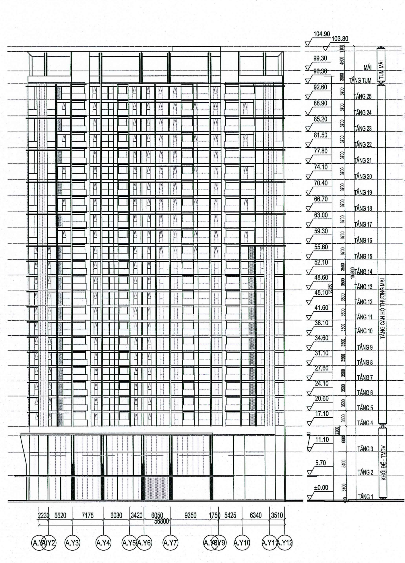
CT2 - MẶT ĐỨNG TRỤC A.Y1-A.Y12
