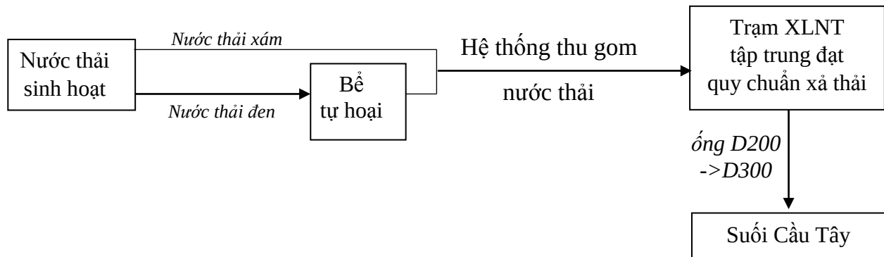
Hình 3. Sơ đồ thu gom nước thải về Trạm XLNT tập trung của Dự án
