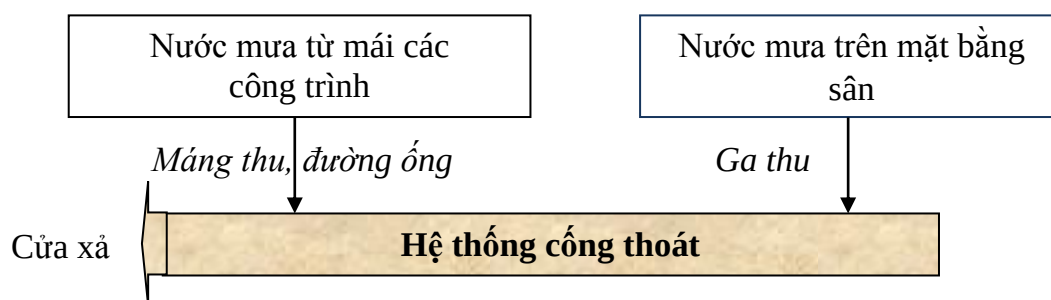
Hình 2. Sơ đồ hệ thống thu gom nước mưa
