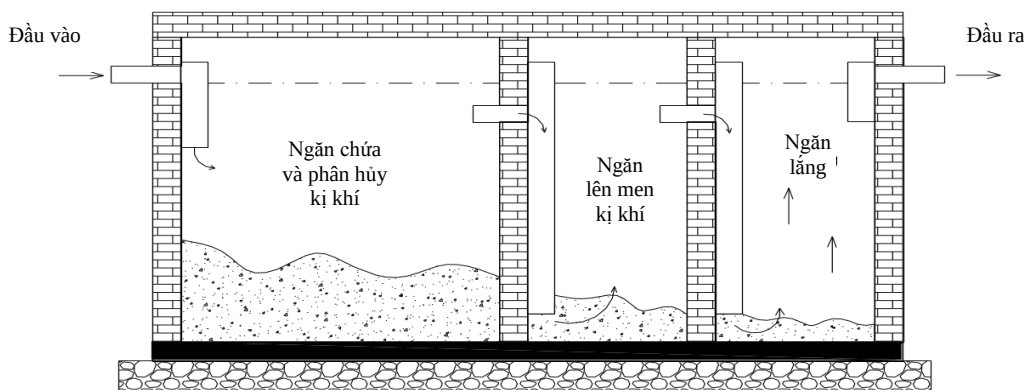
Hình 4. Cấu tạo của bể tự hoại 3 ngăn
