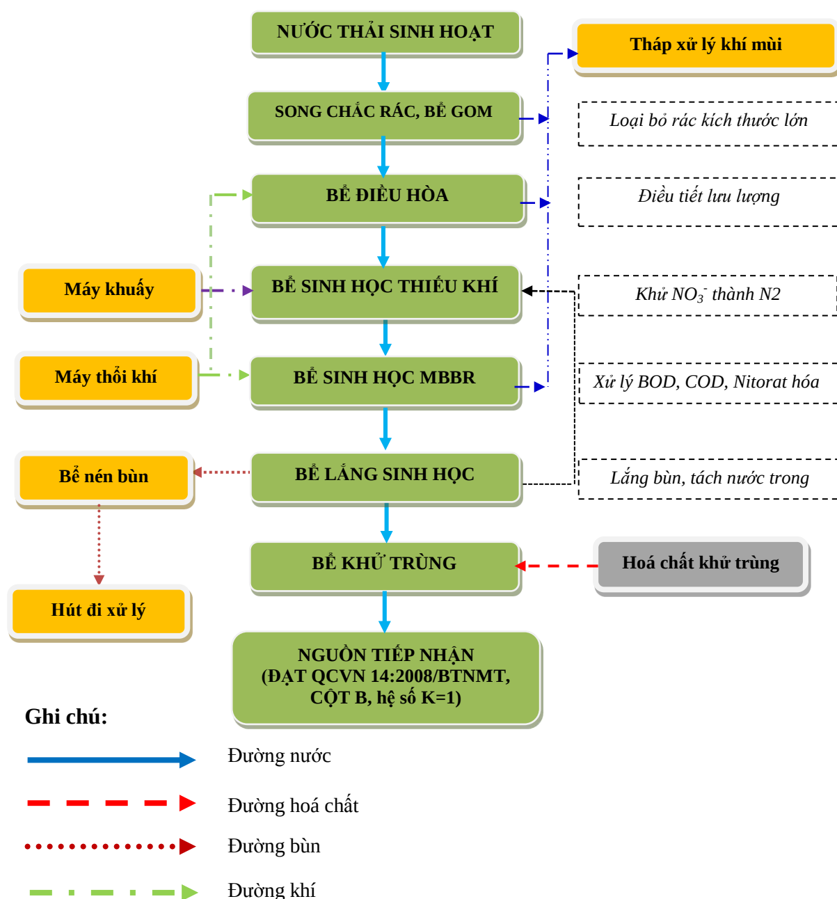
Hình 5. Sơ đồ công nghệ trạm xử lý nước thải 30m 3 /ngày đêm
