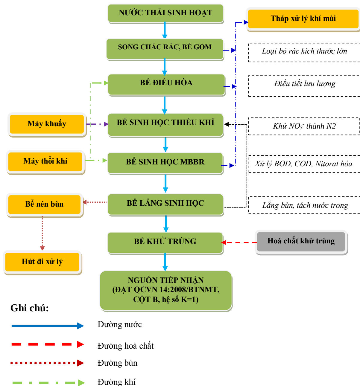
Hình 3. 5. Sơ đồ công nghệ hệ thống xử lý nước thải của dự án
