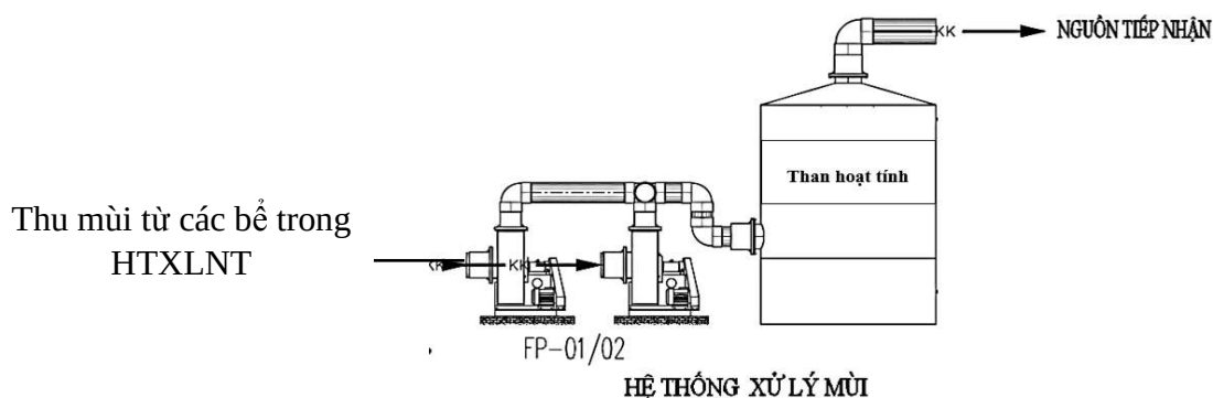
Hình 6. Sơ đồ hệ thống xử lý khí thải từ Trạm XLNT
