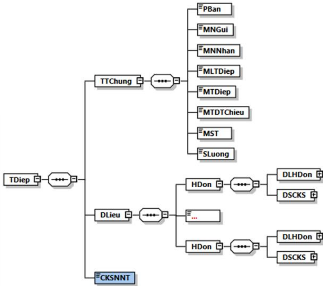
Hình minh họa: Định dạng thông điệp gửi hóa đơn khởi tạo từ máy tính tiền đã cấp mã tới cơ quan thuế.
